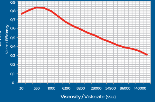
Pump Caharacteristic Graphs / Pompa Karakteristik Grafikleri
