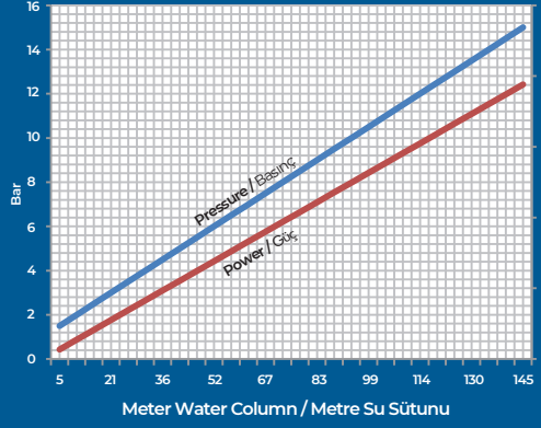
Pump Caharacteristic Graphs / Pompa Karakteristik Grafikleri
